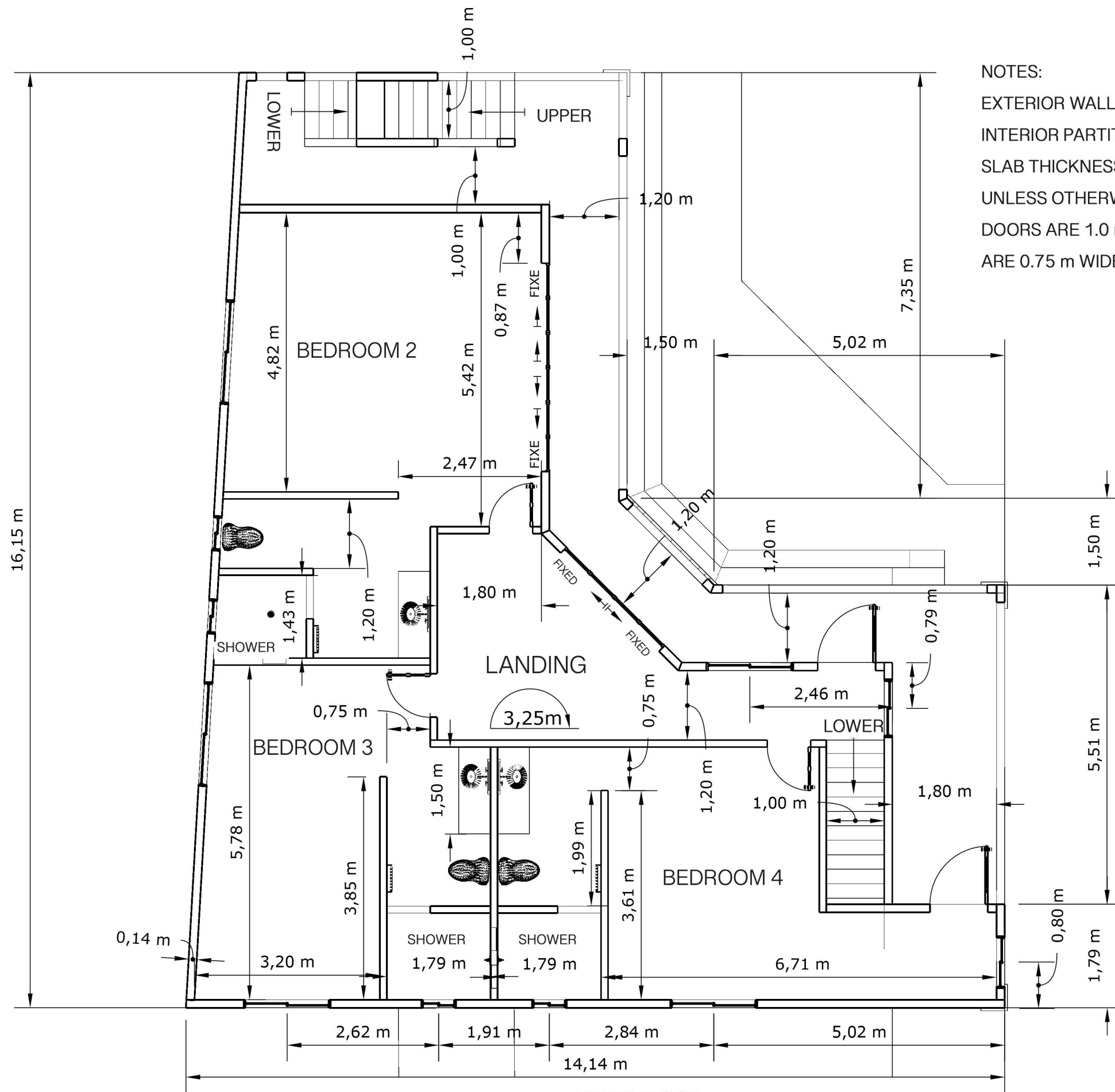
UPPER FLOOR SCALE: 1:75
